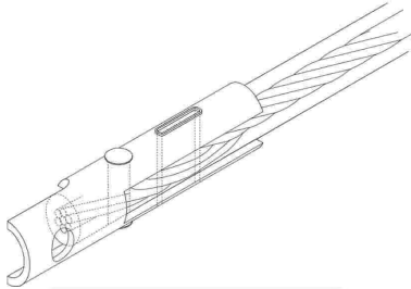
2. Widok boczny – tył
