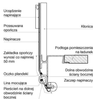
Rysunek 9.3 DOLNA ZAKŁADKA OPOŃCZY
