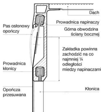
Rysunek 9.2 PROWADNICA OPOŃCZY I ZAKŁADKA GÓRNA
